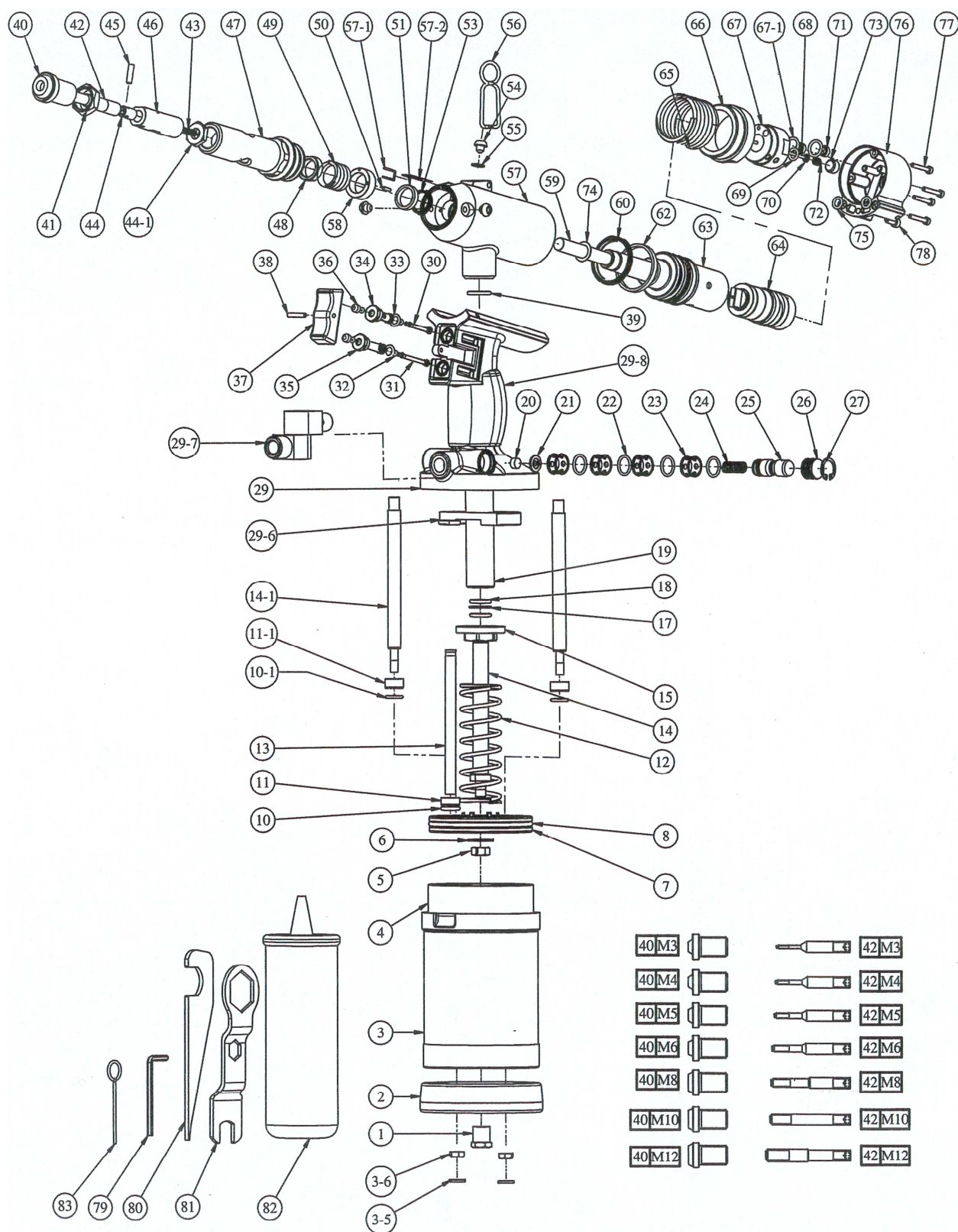
Fig 6 Vue éclatée et pièces détachées de la PI 25
